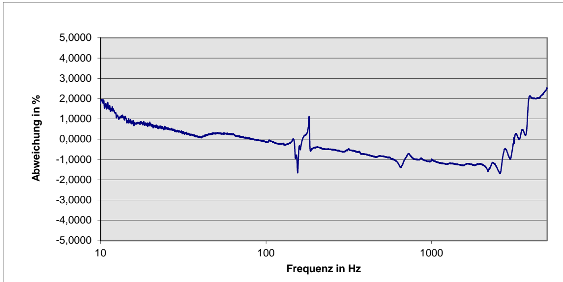
Diagramm Sweep Z-Achse
